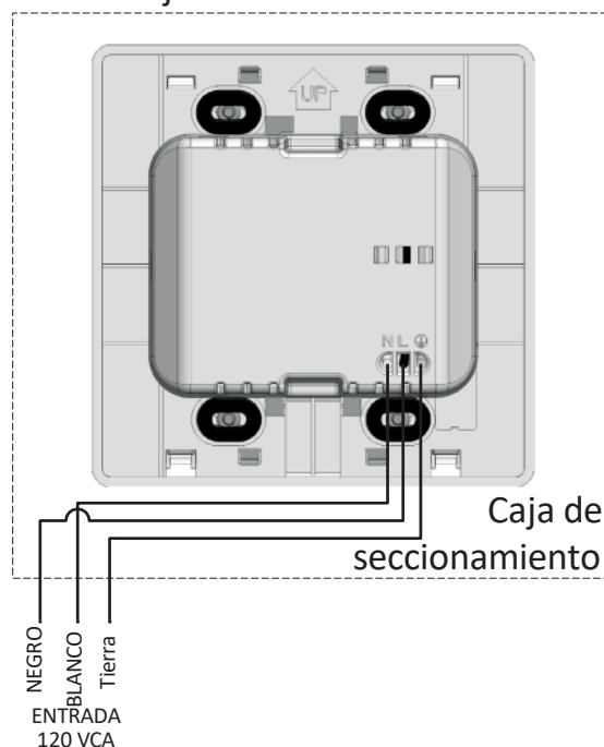
Energía suministrada a la caja de seccionamiento
