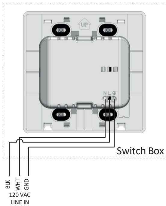
Alimentation électrique vers la boîte de jonction
